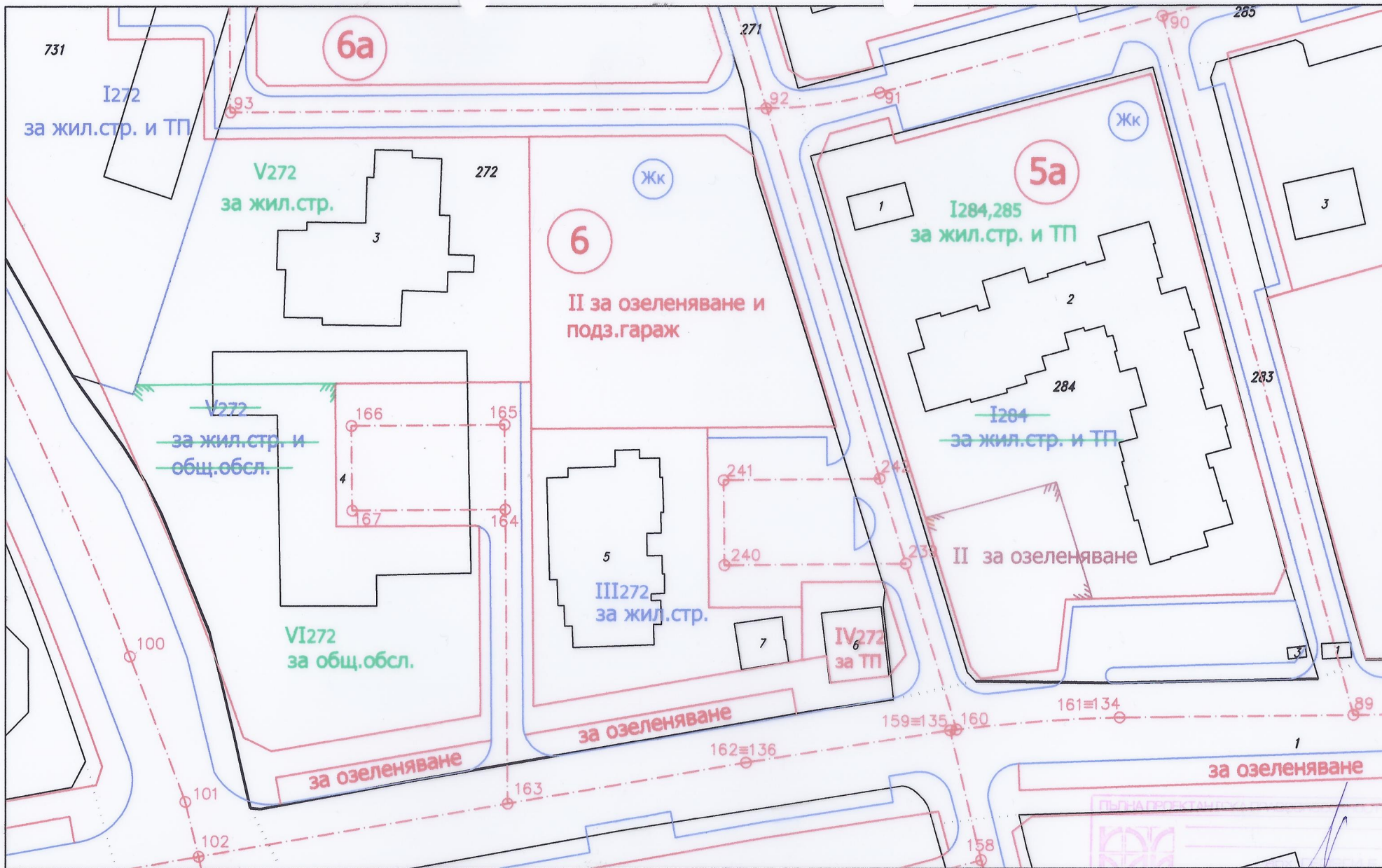
ПРОЕКТ ЗА ИЗМЕНЕНИЕ НА ПЛАН ЗА РЕГУЛАЦИЯ - УПИ V , кв.6 и УПИ I , кв.5а, м.Младост 3, гр.София
